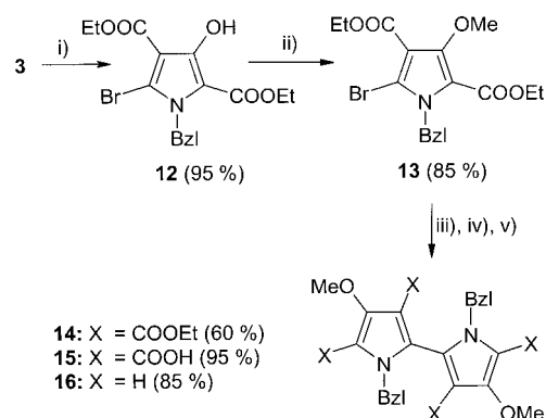
Scheme 3. i) Br_2 ; ii) Me_2SO_4 , acetone, K_2CO_3 , reflux; iii) Cu powder, DMF (trace), 300 °C; iv) KOH, EtOH; v) pyrolysis, 240 °C.
