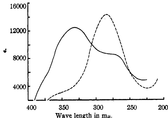
Fig. 4.—Spectra of the ionylidenecyanoacetic acids: ---, \alpha ; —, \beta .
