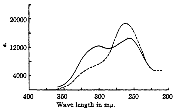
Fig. 5.—Spectra of the ionylideneacetonitriles: ---, \alpha ; —, \beta .
