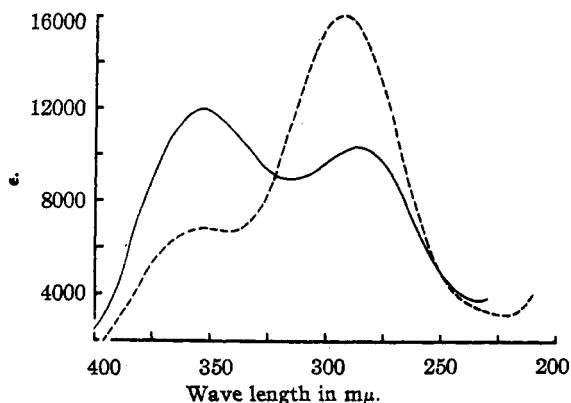
Fig. 3.—Spectra of the methyl ionylidenecyanoacetates: ---, \alpha ; —, \beta .
