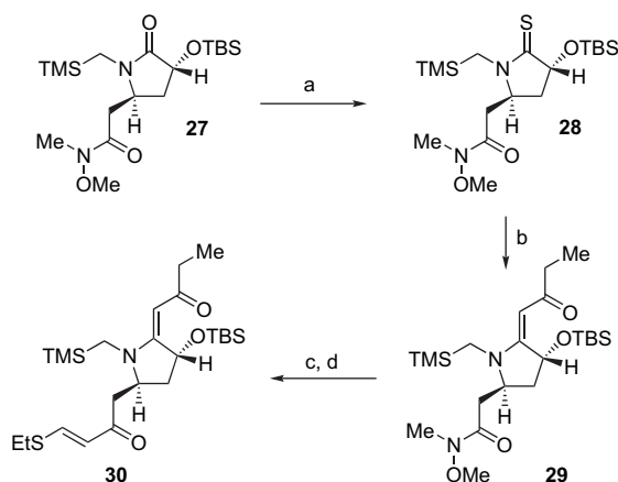
Scheme 7. (a) Lawesson's reagent, PhMe, 23^{\circ}\text{C} , 86%; (b) 1-bromo-2-butanone, 60^{\circ}\text{C} ; Ph 3 P, Et 3 N, CH 2 Cl 2 , 23^{\circ}\text{C} , 52%; (c) HCCMgCl, THF, 23^{\circ}\text{C} ; (d) EtSH, Et 3 N, CH 2 Cl 2 , 23^{\circ}\text{C} , 57% (two steps).
