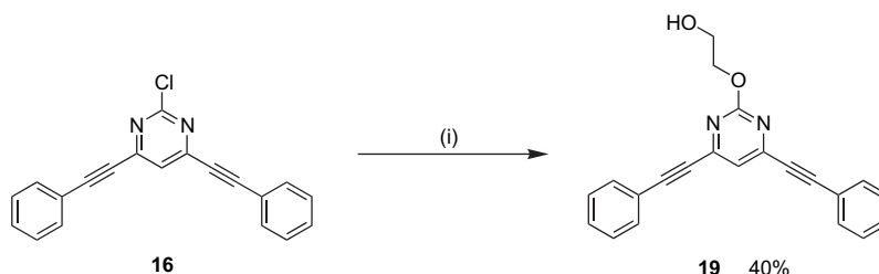
Scheme 5. (i) \text{NaOCH}_2\text{CH}_2\text{OH}/\text{HOCH}_2\text{CH}_2\text{OH} , 15 h, rt.
