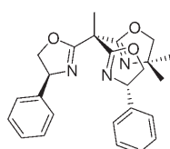
Ph 2 -dm-trisox
