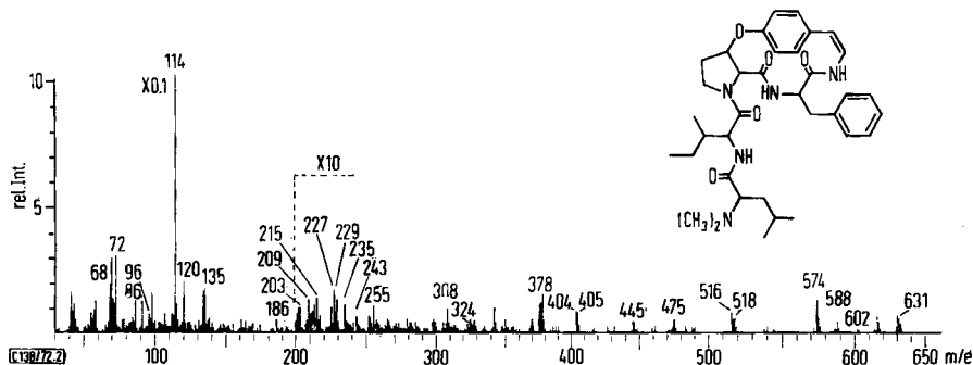
Abbild. 2. Massenspektrum von Amphibin-C
