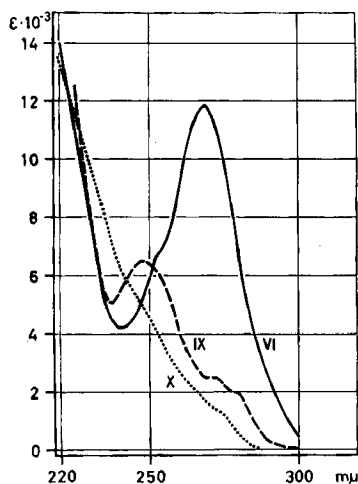
Fig. 2. UV.-Absorptionsspektren in abs. Alkohol
