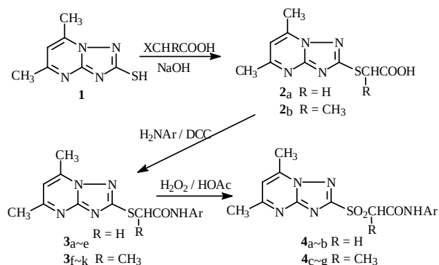
SCHEME 1 (Method A)
