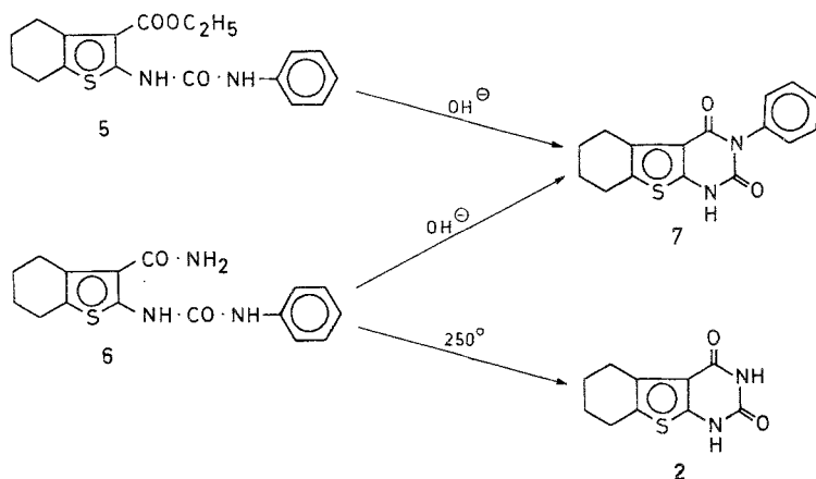
Reaktionsschema 2
