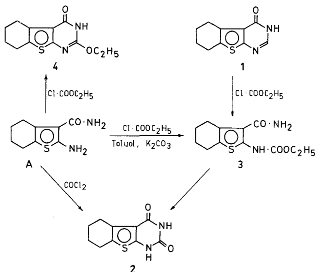
Reaktionsschema 1
