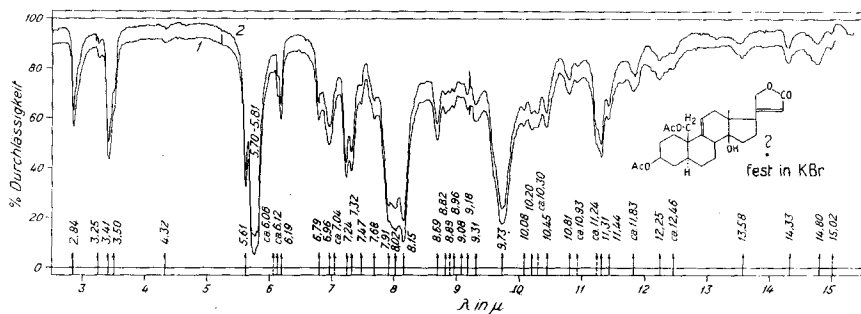
Fig. 22. IR.-Absorptionsspektrum von Di-O-acetyl-pachygenol (XV)
