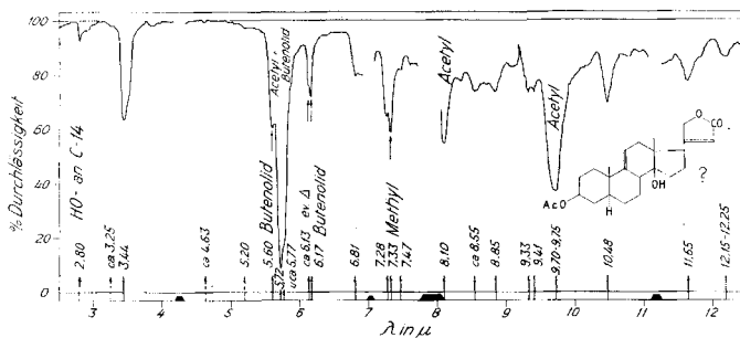
Fig. 19. IR.-Absorptionsspektrum von 3-O-Acetyl-xysmalogenin (VIII) aus Pachycarpus schinzianus
