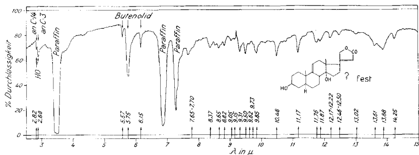
Fig. 18. IR.-Absorptionsspektrum von Xysmalogenin (VII) aus Pachycarpus schinzianus
