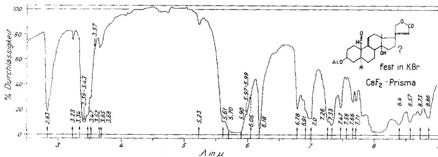
Fig. 21a. IR.-Absorptionsspektrum von O-Acetyl-pachygenin (XIII) Fest in KBr mit \text{CaF}_2 -Prisma 57 ); 3,85 mg pro Pastille
