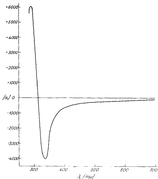
Fig. 23. Optische Rotationsdispersion 63) von Pachygenin (XII) In Dioxan (700–310 m\mu : c = 0,055 ; 320–285 m\mu : c = 0,011 ), 25°
