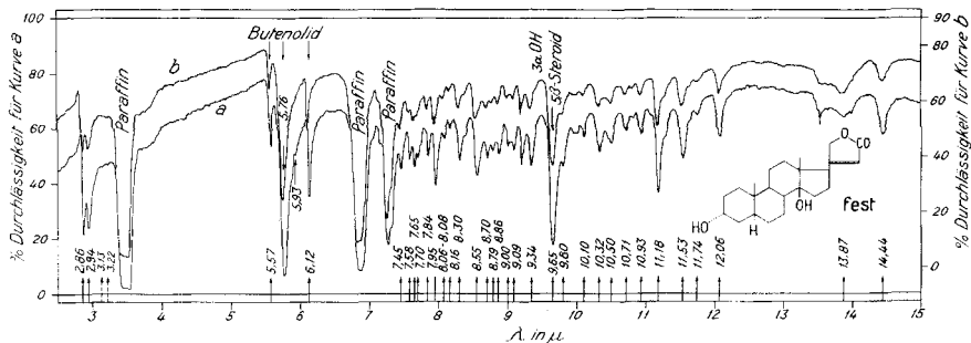
Fig. 17. IR.-Absorptionsspektren von 3-Epi-digitoxigenin (III)
