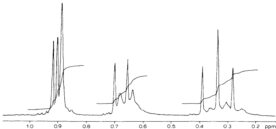
Fig. 2. Gespreizter Bereich der Methylprotonen.
