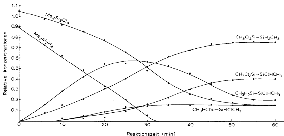
Fig. 3. Äquilibrierung \text{Me}_2\text{Si}_2\text{H}_4/\text{Me}_2\text{Si}_2\text{Cl}_4 bei 90^\circ\text{C} und \text{AlCl}_3 als Katalysator.
