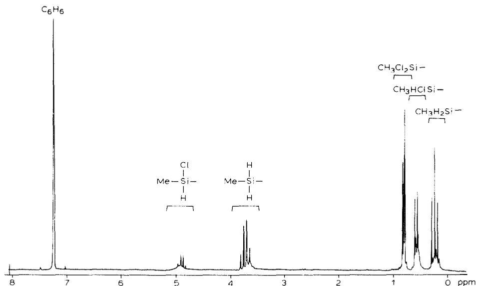
Fig. 1. ^1\text{H} -NMR-Spektrum der Äquilibration von \text{Me}_2\text{Si}_2\text{H}_4 und \text{Me}_2\text{Si}_2\text{Cl}_4 nach 50 min bei 90^\circ\text{C} .
