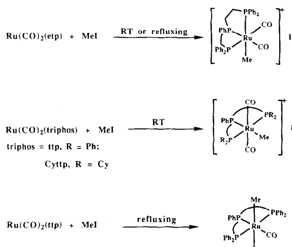
Scheme 2. Reactions of Ru(CO) 2 (triphos) (triphos = etp, ttp, and Cyttp) with MeI in benzene.
