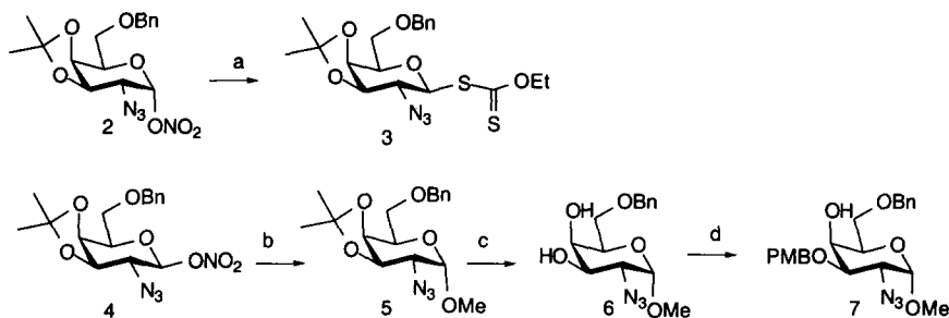
Schéma 1: Réactifs et rendements: a) EtOCSSK, EtOH (88%); b) MeONa, MeOH (64%); c) AcOH aq. à 80%, 80°C (95%); d) 1) Bu 2 SnO, tamis 4Å, CH 3 CN, 80°C, 2) PMB-Br, NBu 4 I, 20°C (90%). (PMB= p-méthoxybenzyl)
