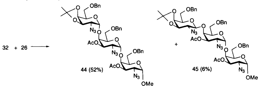
Schéma 13: Réactif: DMTST, CH 2 Cl 2 .
