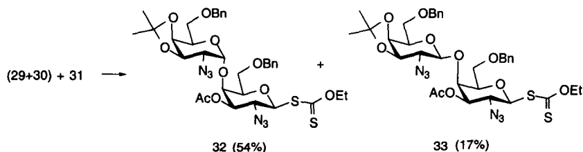
Schéma 10: Réactif: AgOTf, sym -collidine, tamis 4 Å, CH 2 Cl 2 .
