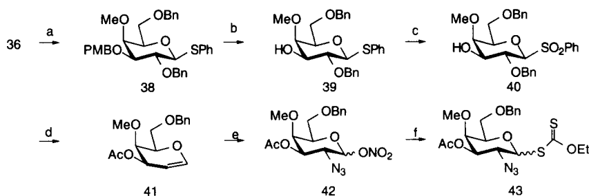
Schéma 12: Réactifs et rendements: a) MeI, NaH, DMF (90%); b) DDQ, CH 2 Cl 2 , H 2 O (93%); c) RuCl 3 , NaIO 4 , CCl 4 , CH 3 CN, H 2 O (94%); d) 1) naphthaléniure de lithium, THF, -78°C; 2) Ac 2 O, DMAP, Pyr. (78%); e) NaN 3 , CAN, -20° C, CH 3 CN, (42 %) rapport α/β 7:3; f) EtO(CS)SK, éthanol (74 %), rapport α/β:2:3.
