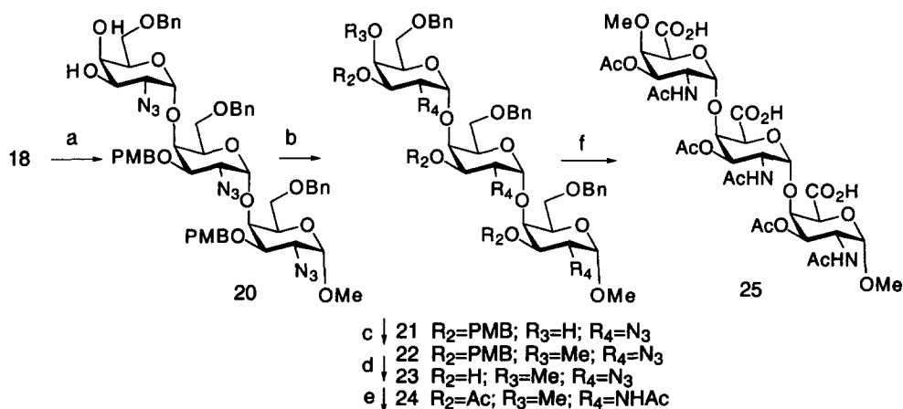
Schéma 5: Réactifs et rendements: a) AcOH aq. à 80%, 80°C (80%); b) 1) Bu 2 SnO, tamis 4Å, CH 3 CN, 80°C, 2) PMB-Br, NBu 4 I, 20°C (90%); c) MeI, NaH, DMF, 81%; d) AcOH aq. à 60%, 130°C (74%); e) 1) NaBH 4 , NiCl 2 , EtOH, 2) Ac 2 O, pyr. (60%); f) 1) H 2 , Pd/C, MeOH (93%); 2) RuCl 3 , NaIO 4 , CCl 4 , CH 3 CN, H 2 O (88%).
