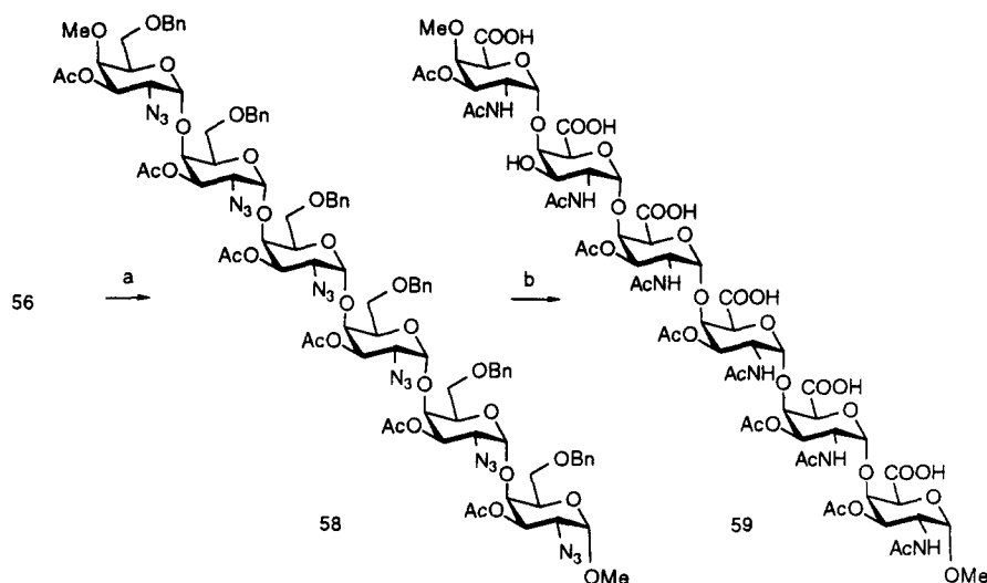
Schéma 18: Réactifs et rendements: a) \text{CH}_3\text{COSH} , \text{CH}_3\text{COSK} , \text{DMF} (65 %); b) 1) \text{H}_2 , \text{Pd/C} , \text{MeOH} ; 2) \text{RuCl}_3 , \text{NaIO}_4 , \text{CCl}_4 , \text{CH}_3\text{CN} , \text{H}_2\text{O} (78%)
