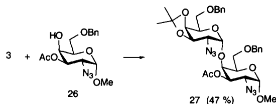
Schéma 7: Réactif: DMTST, CH 2 Cl 2 , 20°C.
