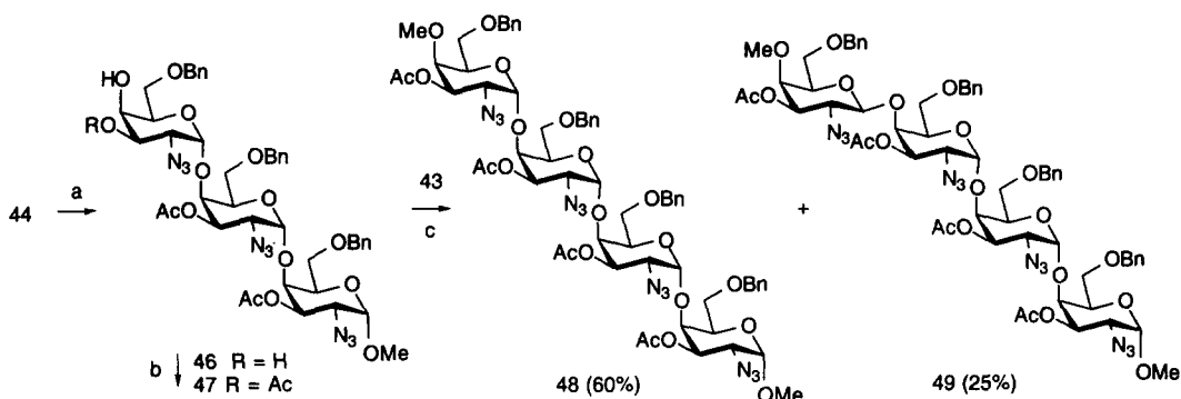
Schéma 14: Réactifs et rendements: a) AcOH aq. à 80%, 80°C (84%); b) 1) Bu 2 SnO, Tamis 4Å, CH 3 CN, 80°C, 2) AcCl, 20°C (97%); c) DMTST, CH 2 Cl 2 .
