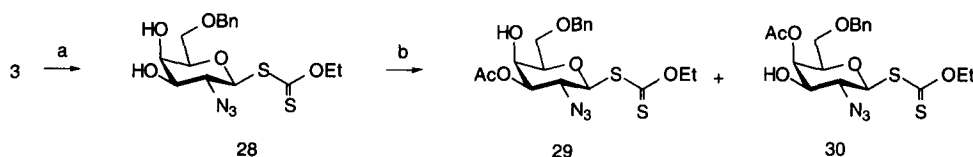
Schéma 8: Réactifs et rendements: a) AcOH aq à 80%, 80°C (93%); b) AcCl, Pyr., -20°C, 29/30 10:3 (88%)
