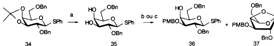
Schéma 11: Réactifs et rendements: a) AcOH aq à 80°C (97%); b) 1) Bu 2 SnO, tamis 4Å, CH 3 CN, 80°C, 2) PMB-Br, NBu 4 I, 20°C 36 : (43%) 37 : (31%); c) 1) Bu 2 SnO, Tamis 4Å, Ph-Me, 80°C, 2) PMB-Br, NBu 4 Br, 100°C 36 : (92%).
