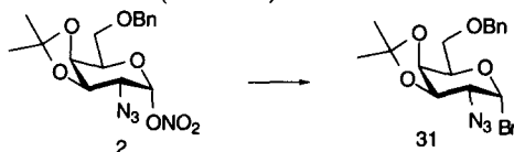
Schéma 9: Réactif: LiBr, CH 3 CN, 20°C.
