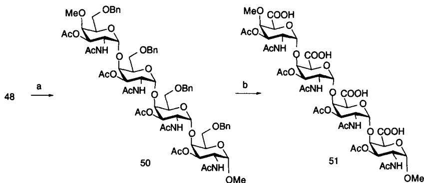
Schéma 15: Réactifs: a) CH 3 COSH, CH 3 COSK, DMF (70 %); b) 1) H 2 , Pd/C, MeOH; 2) RuCl 3 , NaIO 4 , CCl 4 , CH 3 CN, H 2 O (60%)
