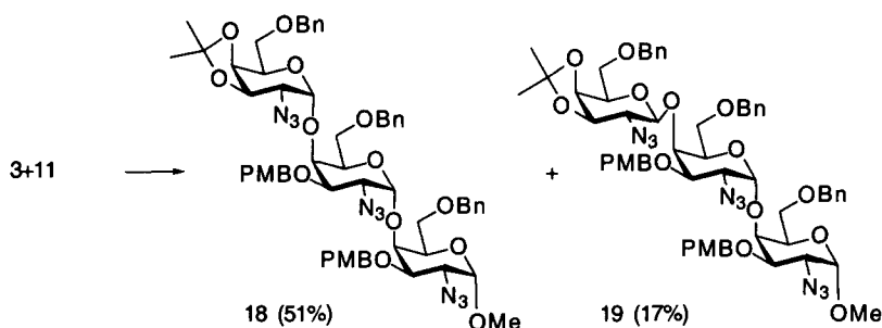
Schéma 4: Réactif: DMTST, CH 2 Cl 2 , 20°C.
