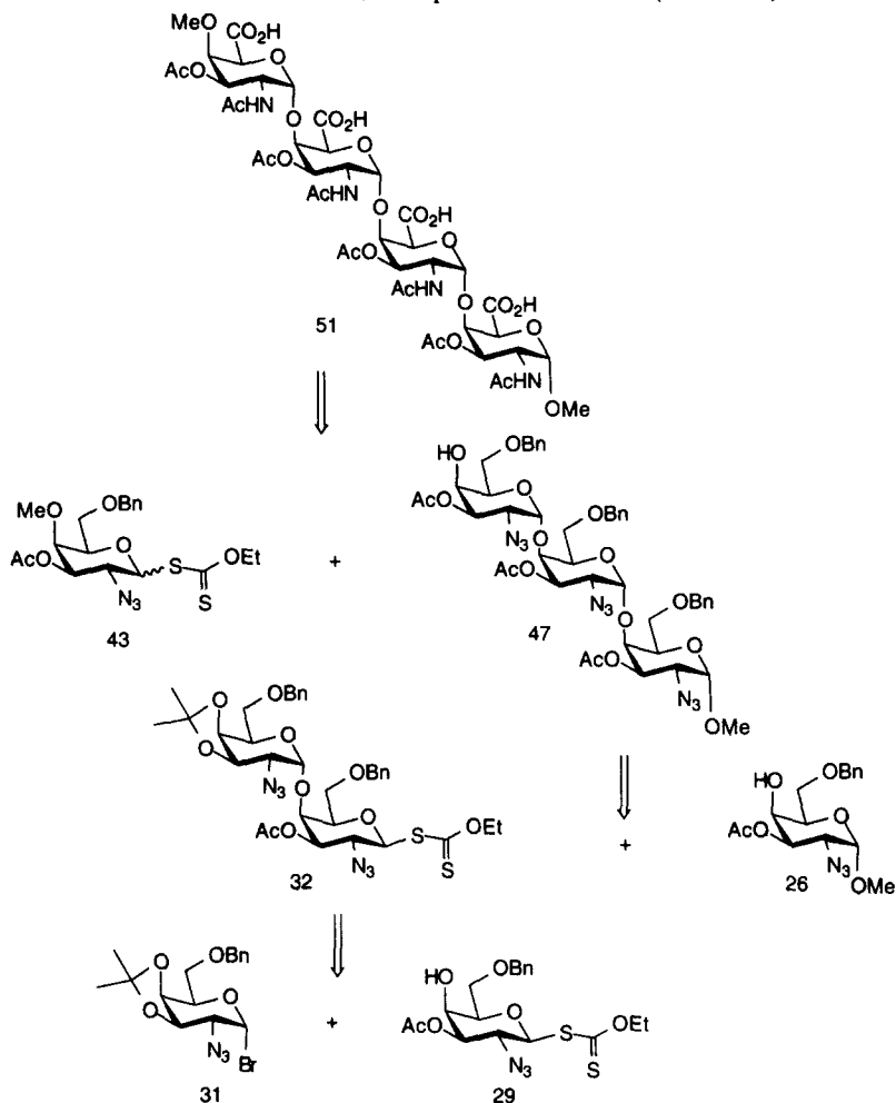
Schéma 6: Rétrosynthèse du tétrasaccharide 51 .
