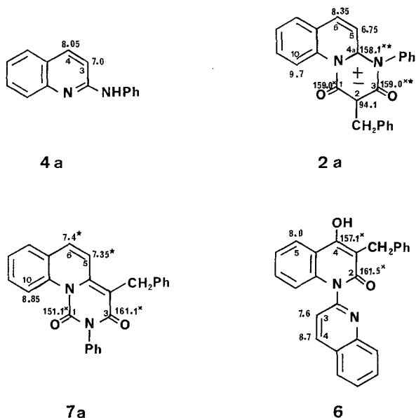
Abb. 2. ^1\text{H} - und ^{13}\text{C} (*)-NMR-Daten; mit * bezeichnete Werte können vertauscht werden
