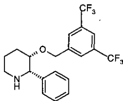
L-733060
