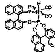
RhH(CO) 2 [(R,S)-BINAPHOS]
