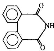
Diphenimide (XVI)
