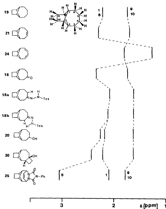
Fig. 1. Vergleich der ^1\text{H} -NMR-Daten der Cyclobutan-Protonen \text{H}-\text{C}(1) und \text{H}-\text{C}(8) mit denjenigen der Protonen \text{CH}_2(9) und \text{CH}_2(10) der untersuchten Tricyclo[5.3.0.0 2,8 ]decane
