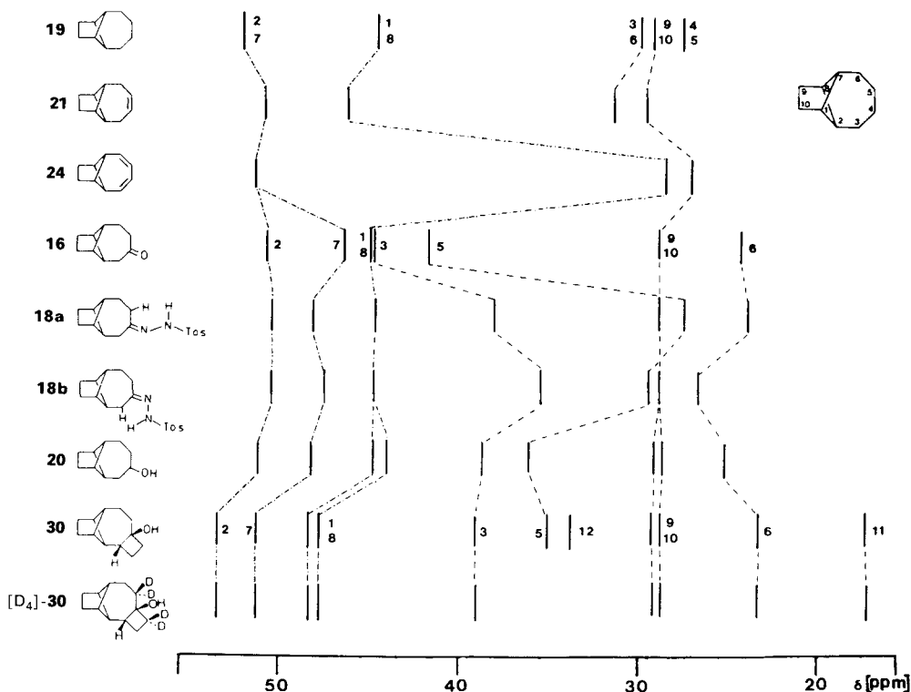
Fig. 2. Vergleich der ^{13}\text{C} -NMR-Daten der untersuchten Tricyclo[5.3.0.0 2,8 ]decane zwischen 15 und 60 ppm
