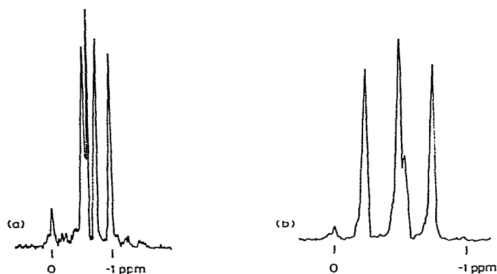
Fig. 2. Spectres RMN de ^{119}\text{Sn} de deutéroalkyltriméthylétaïens. (a) Spectre d'un mélange de III et VII; (b) spectre d'un mélange de III et VI.
