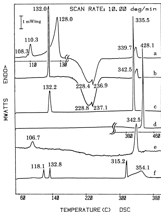
Fig. 1. The DSC curves of KDN, KDN/ \text{KNO}_3 , \text{KNO}_3 and \text{KNO}_2 : (a) KDN; (b) pure KDN; (c) \text{KNO}_3 ; (d) \text{KNO}_2 ; (e) decomposition residue of KDN; (f) \text{KNO}_3/\text{KNO}_2 = 1:1 .
