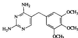
1 Trimethoprim
