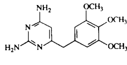
2 Isotrimethoprim
