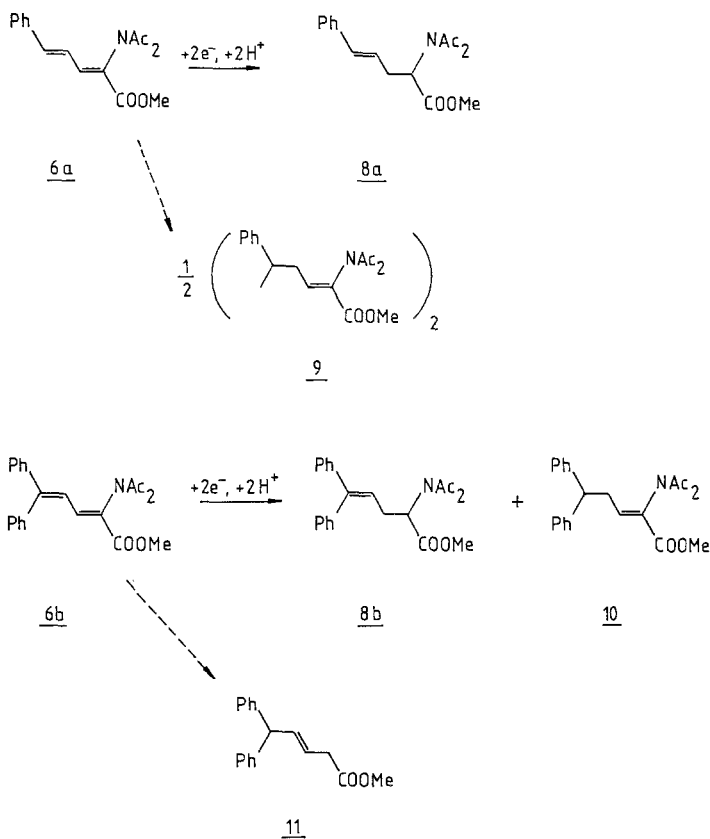
Schema 2. Kathodische Reduktion der N,N-Diacetylmino-2,4-pentadiensäureester 6a und 6b
