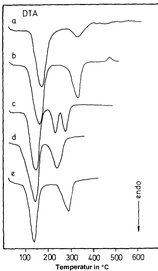
Abbildung 2. DTA-Kurven der thermischen Entwässerung unter quasi-isobaren Bedingungen
