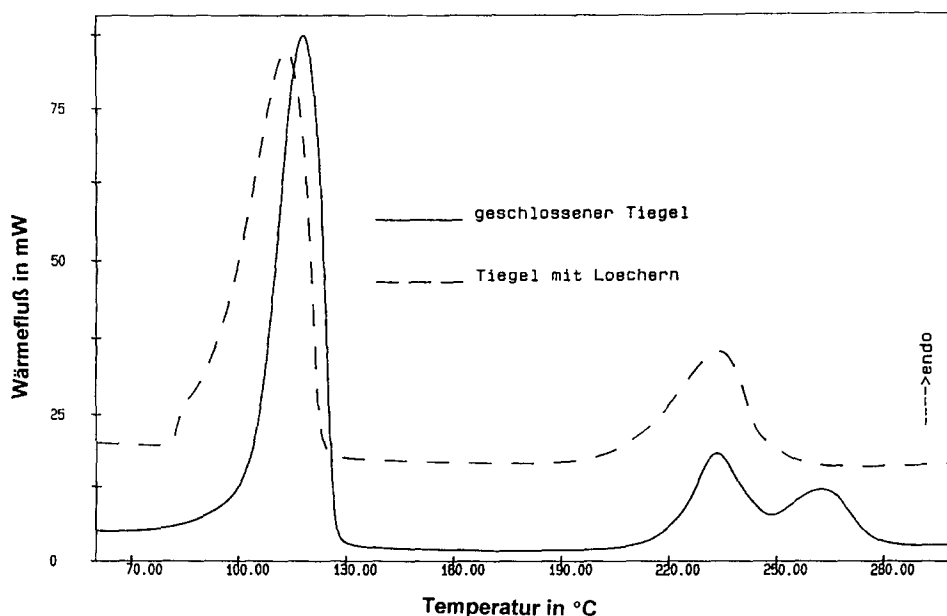
Abbildung 3. DSC-Kurven der thermischen Entwässerung von \text{Fe}_2\text{F}_5 \cdot 7\text{H}_2\text{O}
