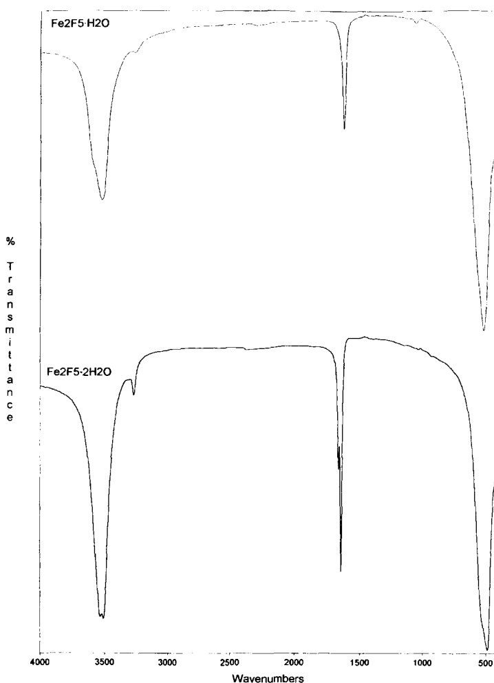
Abbildung 5. Vergleich der IR-Spektren von \text{Fe}_2\text{F}_5 \cdot 2\text{H}_2\text{O} und \text{Fe}_2\text{F}_5 \cdot \text{H}_2\text{O}
