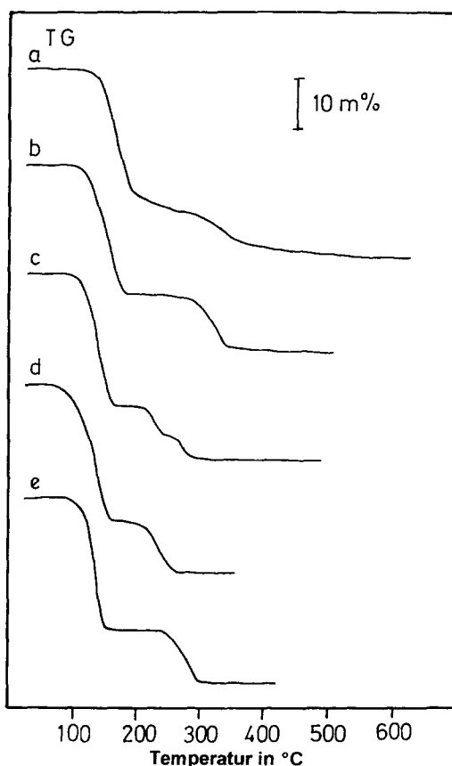
Abbildung 1. TG-Kurven der thermischen Entwässerung unter quasi-isobaren Bedingungen
