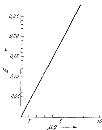
Abb. 1. Eichkurve des 2,6-Dimethylphenol-indophenols. Die Messung wurde auf einem Zeiss-Spektralphotometer PMQ II bei 500 m\mu durchgeführt.
