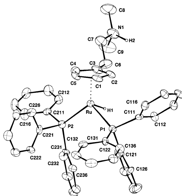
Figure 3. CAMERON view of [(C 5 H 4 CH 2 CH 2 NHMe 2 )-RuH(PPh 3 ) 2 ](BPh 4 )·H 2 O ( 4 ·H 2 O). Selected bond lengths (Å): Ru–H(1), 1.58(13); Ru–P(1), 2.248(2); Ru–P(2), 2.270(2); Ru–C(1), 2.244(7); Ru–C(2), 2.235(8); Ru–C(3), 2.239(7); Ru–C(4), 2.238(8); Ru–C(5), 2.287(8); N(1)–H(2), 1.02(3). Selected bond angles (deg): P(1)–Ru–P(2), 100.75(7); P(1)–Ru–H(1), 80.6(45); P(2)–Ru–H(1), 94.5(46).
