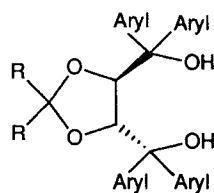
1 ( C_2 -symmetrical)
