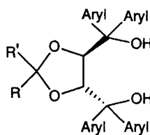
2 ( C_1 -symmetrical)
