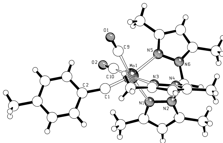
Fig. 1. Molecular structure of [tpb'(CO)_2Mo\equiv CC_6H_4Me-4] ( 4b ). Important bond distances (Å) and angles ( ^\circ ) with estimated S.D. in parentheses: 4b : Mo1–C1 1.804(4), Mo1–C9 1.987(4), Mo1–C10 1.987(4), Mo1–N1 2.218(3), Mo1–N3 2.212(3), Mo1–N5 2.306(3), C1–C2 1.449(5), C9–O1 1.145(5), C10–O2 1.140(5); Mo1–C1–C2 163.1(3), Mo1–C9–O1 176.9(4), Mo1–C10–O2 176.3(4). 6 : W1–C1 1.829(3), W1–C9 1.985(4), W1–C10 1.994(4), W1–N1 2.210(3), W1–N3 2.288(3), W1–N5 2.203(3), C1–C2 1.448(4), C9–O1 1.159(5), C10–O2 1.146(5); W1–C1–C2 163.2(3), W1–C9–O1 177.6(4), W1–C10–O2 176.3(4).
