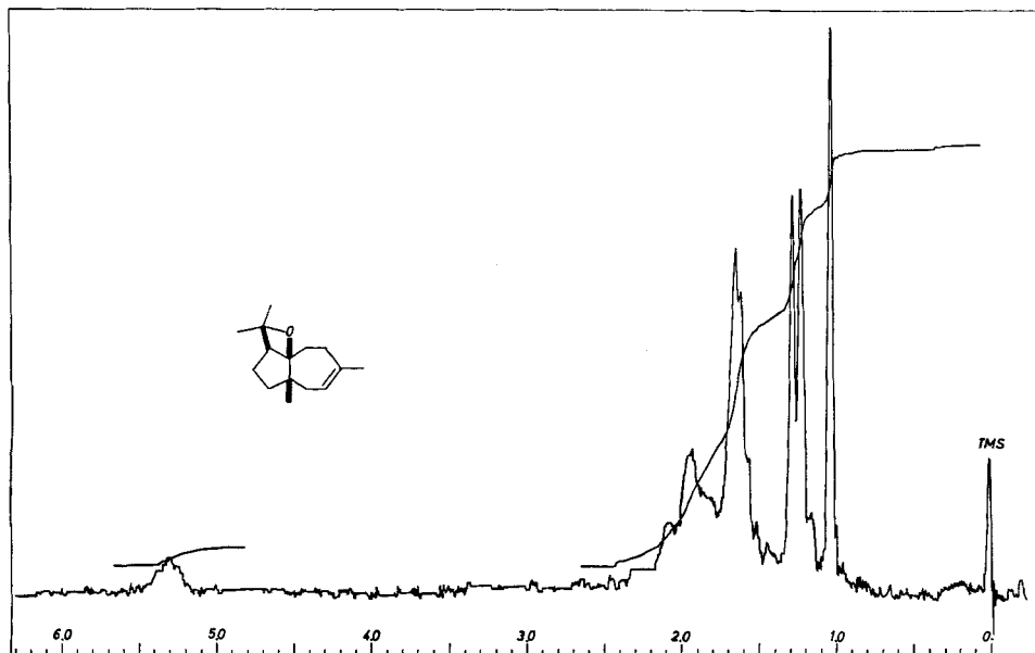
Fig. 2. Spectre de RMN. du «carotol-éther» 12 (CDCl 3 + CCl 4 )
