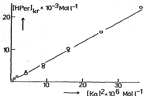
Fig. 2. Kritische Hydroperoxidkonzentration [\text{HPer}]_{\text{kr}} als Funktion von [\text{Ka}]^2 für [\text{Cyclohexen}] = 1 (○); 2 (X) und 3 (□) \text{Mol l}^{-1} .
