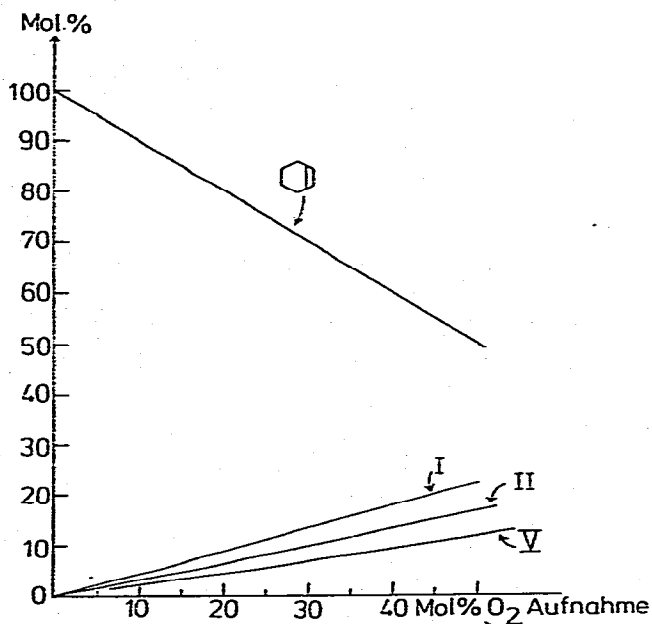
Fig. 5. Produktzusammensetzung der katalytischen Oxidation von Cyclohexen, gelöst in Benzol bei 60 °C mit dem Katalysator IrCl(CO)(PPh 3 ) 2 , als Funktion der Mol% O 2 aufgenommen. Die Werte wurden erhalten mit [Ka] = 2, 3 und 4 mMol l -1 und [Cyclohexen] = 2, 3, 4 und 9.86 Mol l -1 (reines Cyclohexen); I: Cyclohexen-2-on-1; II: Cyclohexen-2-ol-1; V: nicht identifizierte Produkte.
