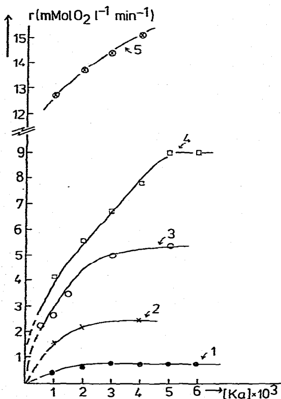
Fig. 3. Geschwindigkeit r der \text{O}_2 -Aufnahme ( \text{mMol O}_2 \text{ l}^{-1} \text{ min}^{-1} ) in den ersten 30 Minuten der Oxidation von Cyclohexen, gelöst in Benzol bei 60^\circ \text{C} ; mit dem Katalysator \text{IrCl}(\text{CO})(\text{PPh}_3)_2 als Funktion der [\text{Ka}] und [\text{Cyclohexen}] ; p(\text{O}_2) = 400 \text{ Torr} . Die Kurven 1, 2, 3 und 4 entsprechen einer [\text{Cyclohexen}] = 1, 2, 3, 4 \text{ Mol l}^{-1} ; Kurve 5: reines Cyclohexen (Konz. \approx 9.86 \text{ Mol l}^{-1} ); [\text{HPer}] beim Start: 25 \text{ mMol l}^{-1} .
