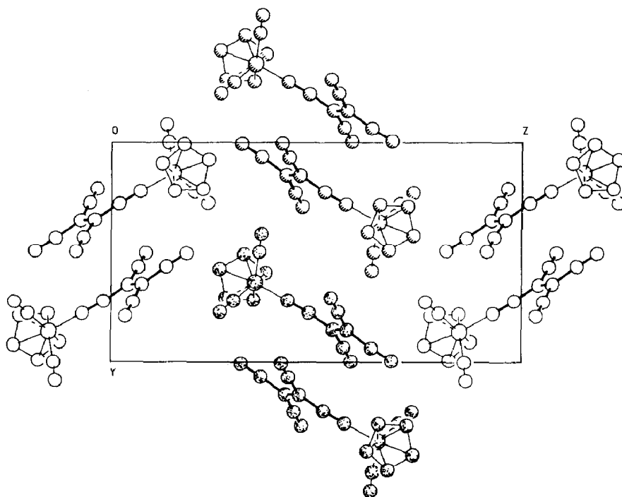
Fig. 2. Darstellung der Festkörperstruktur von 1 (nächstbenachbarte TCNE-Paare sind jeweils gleich gekennzeichnet).
