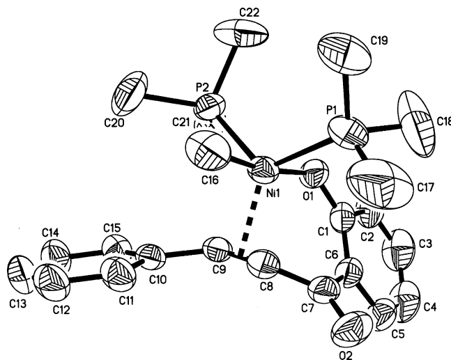
Figure 3. Molecular structure 14 of complex 2 and selected bond parameters (Å, deg): \text{Ni}-\text{O}(1) 1.9359(18), \text{Ni}-\text{C}(8) 2.075(3), \text{Ni}-\text{C}(9) 2.127(2), \text{Ni}-\text{C}(16) 1.975(3), \text{Ni}-\text{P}(1) 2.2443(10), \text{Ni}-\text{P}(2) 2.2477(10), \text{C}(6)-\text{C}(7) 1.473(4), \text{C}(7)-\text{C}(8) 1.468(4), \text{C}(8)-\text{C}(9) 1.393(4), \text{C}(9)-\text{C}(10) 1.476(3), \text{C}(1)-\text{C}(6) 1.412(4), \text{C}(1)-\text{O}(1) 1.308(3); \text{O}(1)-\text{Ni}-\text{C}(16) 170.77(12), \text{O}(1)-\text{Ni}-\text{C}(9) 91.22(9), \text{C}(16)-\text{Ni}-\text{C}(9) 97.19(12), \text{O}(1)-\text{Ni}-\text{P}(1) 88.88(6), \text{C}(8)-\text{Ni}-\text{P}(1) 104.76(8), \text{C}(16)-\text{Ni}-\text{P}(2) 89.87(12), \text{P}(1)-\text{Ni}-\text{P}(2) 117.99(4), \text{C}(7)-\text{C}(8)-\text{C}(9) 123.2(2), \text{O}(1)-\text{Ni}-\text{C}(8) 95.05(9), \text{C}(16)-\text{Ni}-\text{C}(8) 93.89(13), \text{C}(8)-\text{Ni}-\text{C}(9) 38.69(10), \text{C}(16)-\text{Ni}-\text{P}(1) 86.65(12), \text{O}(1)-\text{Ni}-\text{P}(2) 85.11(6), \text{C}(9)-\text{Ni}-\text{P}(2) 98.57(7), \text{C}(8)-\text{C}(9)-\text{C}(10) 125.9(2).
