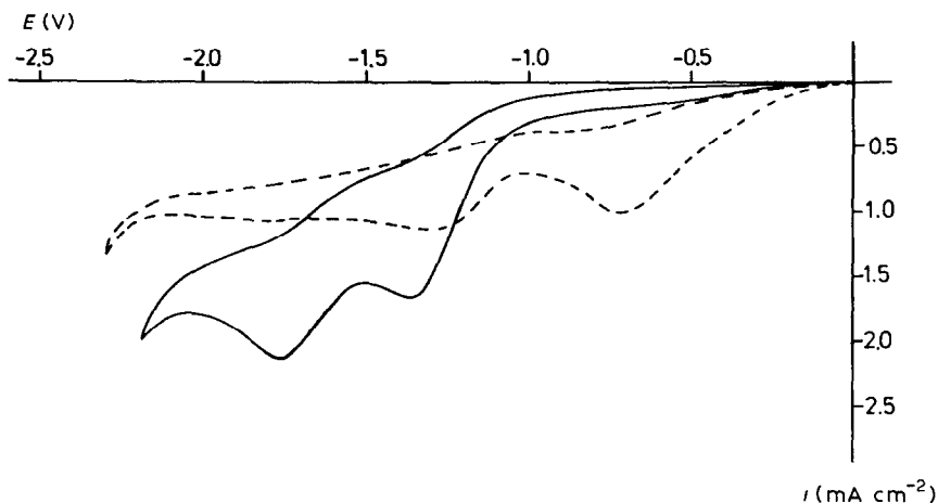
Fig. 1. CV von 1a (—) und 1b (---) an Pt in 0.3 M [Bu 4 N]Br/CH 2 Cl 2 , Bezugselektrode: ges. Kalomel-Elektrode, \nu 50 mV s -1 , T -30°C.
