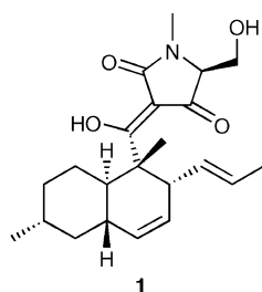
Fig. 1 Equisetin 1 .
