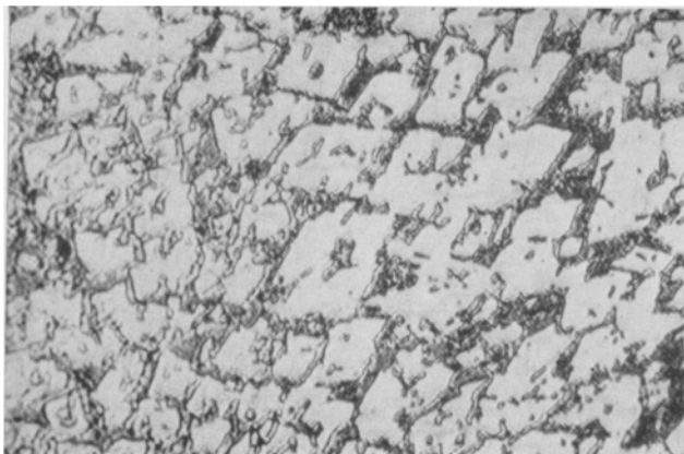
Abb. 4. Gefüge von \text{Ta(3)Si} . \times 600
