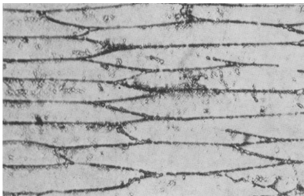
Abb. 3. Gefüge von \text{Ta}_2\text{Si} . \times 600
