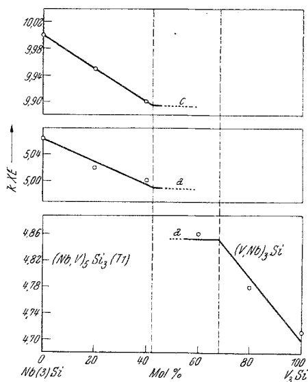
Abb. 9. Verlauf der Gitterkonstanten in der Mischreihe \text{V}_3\text{Si} —Nb(3)Si
