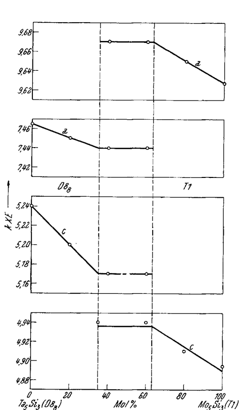
Abb. 8. Verlauf der Gitterkonstanten in der Mischreihe \text{Ta}_5\text{Si}_3 ( D 8_8 )— \text{Mo}_5\text{Si}_3 ( T 1 ) bei 1800° C
