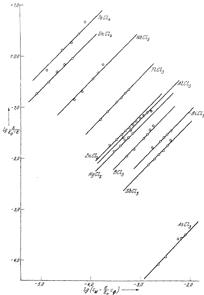
Abb. 6. Gleichgewichtsgerade für einfache Koordination zu einkernigen Komplexen
