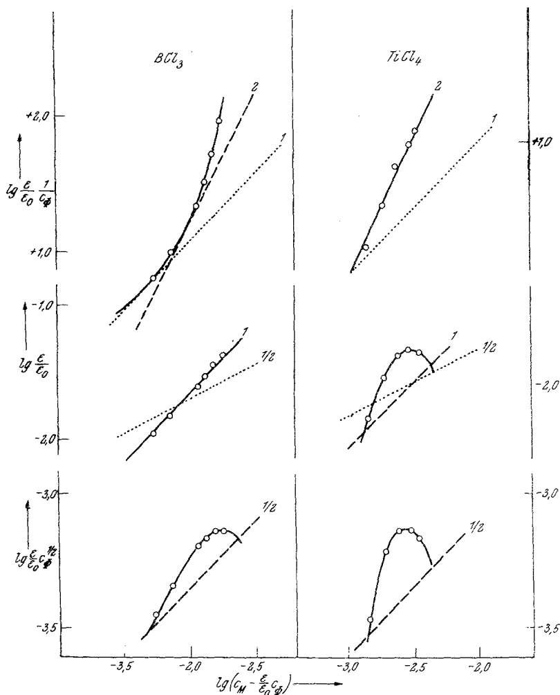
Abb. 5. Identifizierung der vorliegenden Gleichgewichte, gezeigt an zwei charakteristischen Beispielen. Beim \text{BCl}_3 ergibt sich lineare Abhängigkeit zwischen \log \frac{\varepsilon}{\varepsilon_0} und \log \left( c_M - \frac{\varepsilon}{\varepsilon_0} \cdot c_F \right) , beim \text{TiCl}_4 dagegen mit dem Quotienten \log \frac{\varepsilon}{\varepsilon_0} \cdot \frac{1}{c_F} und Steigung 2. Das entspricht einfacher Koordination zu einkernigen bzw. einfacher Koordination zu zweikernigen Komplexen, ohne überlagerte Dissoziation der Ionenpaare
