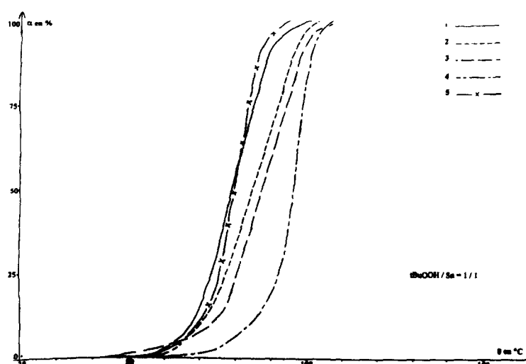
Fig. 1. Degré d'avancement de la réaction de l'hydroperoxyde de t-butyle avec les thioorganostanniques 1 à 5 en fonction de la température.
