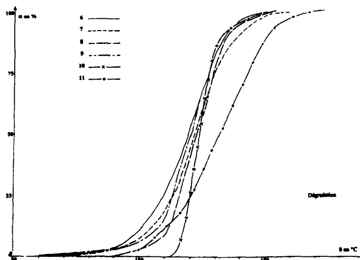
Fig. 4. Degré d'avancement de la réaction de l'hydroperoxyde de t-butyle avec les produits de dégradation des thioorganostanniques 6 à 11 en fonction de la température.
