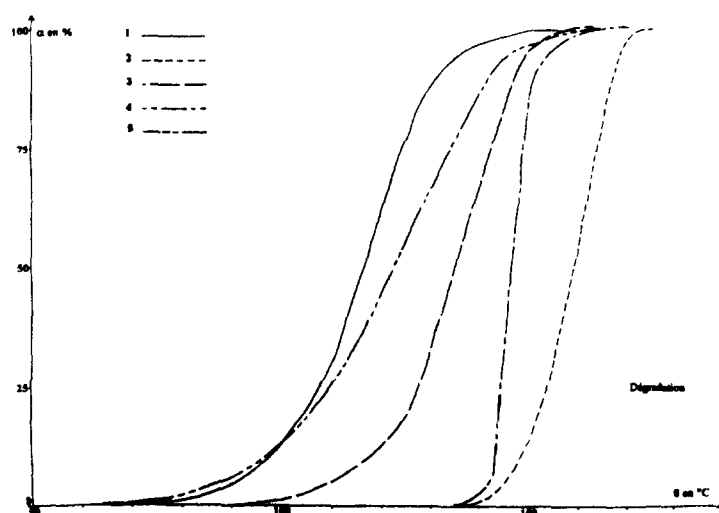
Fig. 3. Degré d'avancement de la réaction de l'hydroperoxyde de t-butyle avec les produits de dégradation des thioorganostanniques 1 à 5 en fonction de la température.
