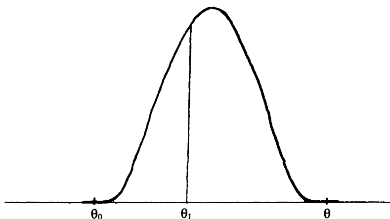
Fig. 5. Thermogramme représentant un endotherme de décomposition.
