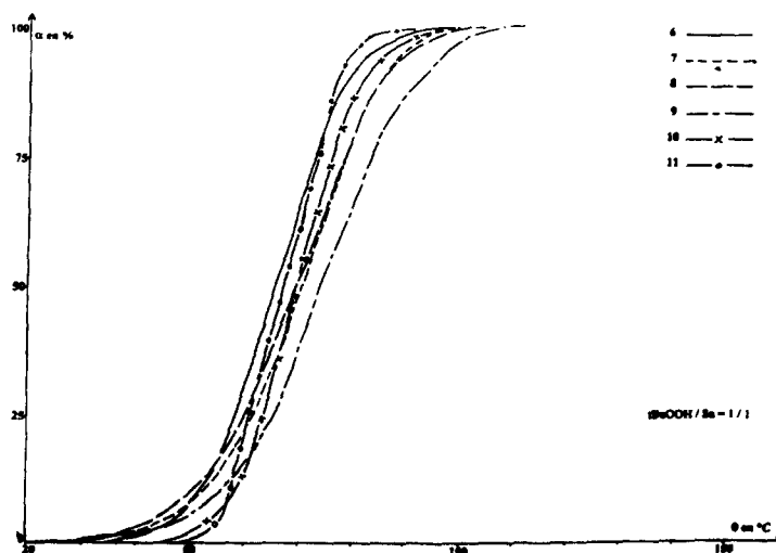
Fig. 2. Degré d'avancement de la réaction de l'hydroperoxyde de t-butyle avec les thioorganostanniques 6 à 11 en fonction de la température.
