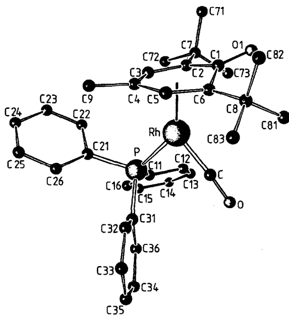
Fig. 1. Ansicht und Atombezeichnung des Moleküls I.
