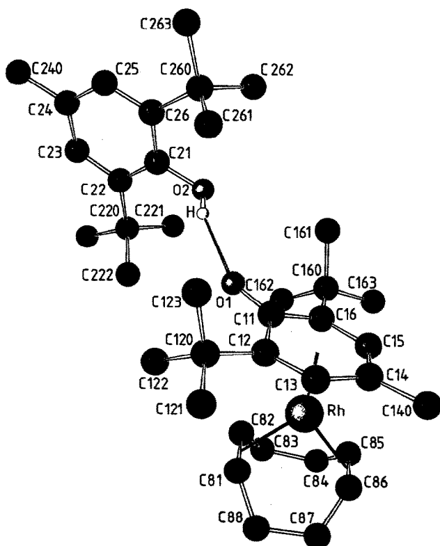
Fig. 2. Ansicht und Atombezeichnung des Moleküls IV \cdot C_{15}H_{24}O .
