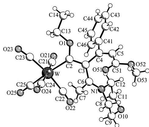
Fig. 1. Molecular structure of carbiminium carbonyltungstate (1Z)- 5a . Selected bond distances (Å) and angles ( ^\circ ): W–C2 2.292(5), C2–O1 1.355(6), C2–C3 1.418(7), O1–C13 1.441(7), C13–C14 1.490(9), C3–C6 1.463(7), C3–C4 1.499(8), C4–C5 1.328(8), C5–C51 1.466(8), C51–O51 1.212(7), C51–O52 1.324(7), O52–C53 1.436(7), C6–N1 1.312(7), C6–C7 1.491(8), N1–C8 1.483(7), N1–C12 1.482(8), C8–C9 1.472(11), C9–O10 1.413(12), O10–C11 1.420(9), C11–C12 1.494(9), O1–C2–C3 106.1(5), O1–C2–W 124.5(4), C3–C2–W 127.7(4), C2–O1–C13 123.8(4), O1–C13–C14 108.7(5), C2–C3–C4 120.4(5), C2–C3–C6 120.8(5), C4–C3–C6 118.8(5), C5–C4–C41 117.9(5), C3–C4–C5 123.8(5), C3–C4–C41 118.1(5), C4–C41–C42 121.0(6), C4–C41–C46 121.4(5), C4–C5–C51 128.9(6), C5–C51–O51 126.4(6), C5–C51–O52 111.6(6), O51–C51–O52 122.0(6), C51–O52–C53 117.5(5), C3–C6–N1 121.0(5), C3–C6–C7 120.2(5), N1–C6–C7 118.5(5), C6–N1–C8 124.6(6), C6–N1–C12 125.3(5), C8–N1–C12 110.1(5), N1–C8–C9 111.1(6), C8–C9–O10 114.2(9), C9–O10–C11 109.1(7), O10–C11–C12 110.4(7), C11–C12–N1 111.1(6).
