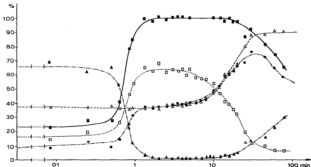
Fig. 1. —■— Rdt. (%) global des énoxysilanes par rapport à la butanone initiale; .....□..... Rdt. (%) en triméthylsiloxy-2 butène-1 (A) par rapport à la butanone initiale; - - - ● - - - Rdt. (%) en triméthylsiloxy-2 butène-2 (B) par rapport à la butanone initiale; - - - Δ - - - % relatif de B/(A + B); - - - ▲ - - - % de butanone restante.
