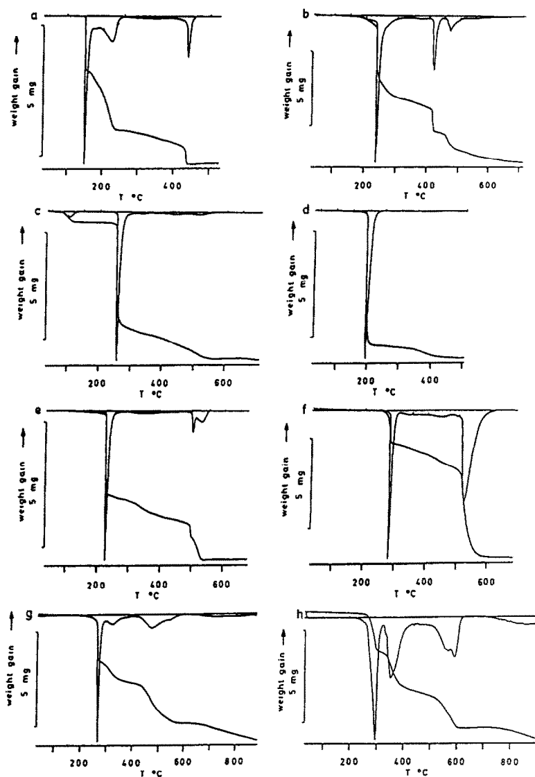
Fig. 2. TG curves for: (a) \text{VO(PTO)}_2 ; (b) \text{Cr(PTO)}_3 ; (c) \text{Mn(PTO)}_2 \cdot \text{H}_2\text{O} ; (d) \text{Fe(PTO)}_3 ; (e) \text{Co(PTO)}_2 ; (f) \text{Ni(PTO)}_2 ; (g) \text{Cu(PTO)}_2 ; and (h) \text{Zn(PTO)}_2 .
