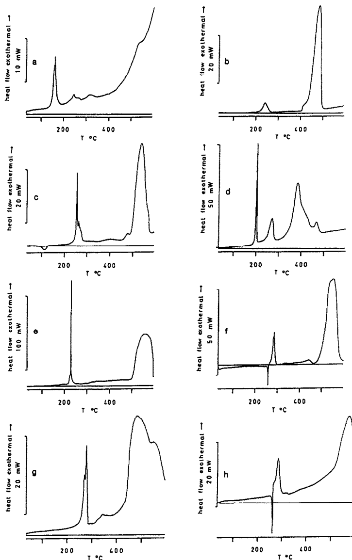
Fig. 3. DSC curves for: (a) \text{VO(PTO)}_2 ; (b) \text{Cr(PTO)}_3 ; (c) \text{Mn(PTO)}_2 \cdot \text{H}_2\text{O} ; (d) \text{Fe(PTO)}_3 ; (e) \text{Co(PTO)}_2 ; (f) \text{Ni(PTO)}_2 ; (g) \text{Cu(PTO)}_2 ; and (h) \text{Zn(PTO)}_2 .
