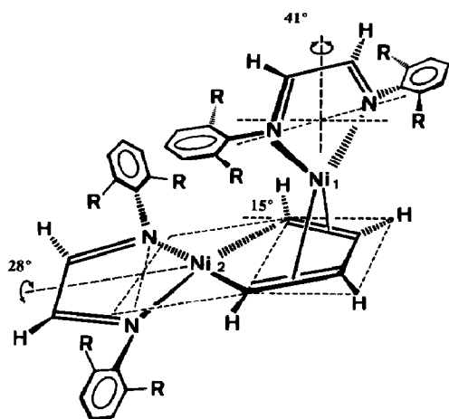
Fig. 1. Schematische Darstellung der Komplexstruktur von 3.
