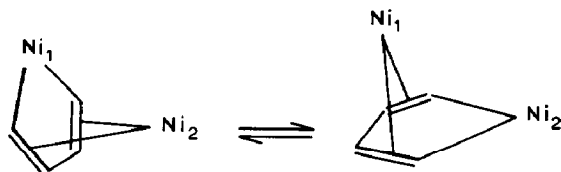
Fig. 2. Austausch der Bindungsverhältnisse von \text{Ni}^0 und \text{Ni}^{\text{II}} bei erhöhter Temperatur.
