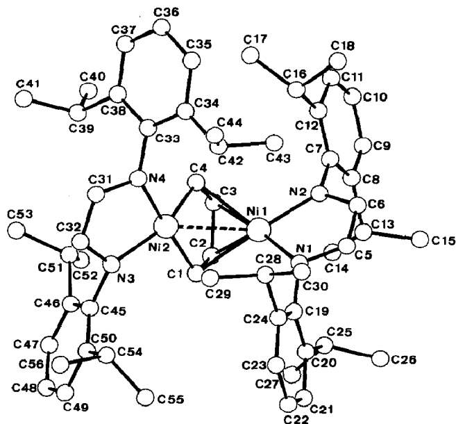
Fig. 3. Kristallstruktur von \{[(^i\text{Pr}_2\text{Ph})_2\text{dad}]\text{Ni}_2(\text{C}_4\text{H}_4)\} (3). Ausgewählte Bindungsabstände (Å) und -winkel ( ^\circ ): Ni(1)–Ni(2) 2.607(1), Ni(1)–C(1) 2.041(4), Ni(1)–C(2) 2.054(4), Ni(1)–C(3) 2.033(4), Ni(1)–C(4) 2.107(4), Ni(2)–C(1) 1.887(4), Ni(2)–C(4) 1.855(4), C(1)–C(2) 1.392(5), C(2)–C(3) 1.417(6), C(3)–C(4) 1.403(5), N(1)–Ni(1)–N(2) 84.1(1), N(3)–Ni(2)–N(4) 84.0(1), C(1)–Ni(2)–C(4) 82.2(2), C(1)–C(2)–C(3) 111.0(3), C(2)–C(3)–C(4) 112.8(3).
