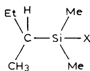
( 5 ; X = Cl, OSO 2 CF 3 )
