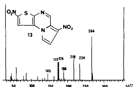
Fig. 1. Spectre de masse de la dinitro-2,6 pyrrolo[1,2-a]thiéo[2,3-e]pyrazine 13 .
