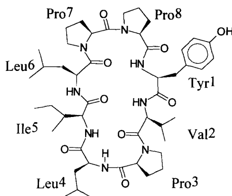
axinastatin 5
