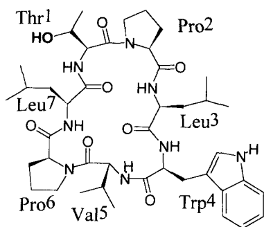
axinastatin 4
