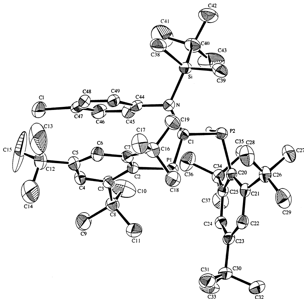
Fig. 2. Molecular structure of \text{Mes}^*\text{P}=\text{C}(\text{PHMes}^*)\text{NAr}(\text{SiMe}_2\text{Bu}) ( 2 ). Selected bond lengths (Å) and angles (°): \text{P}(1)\text{--C}(1) 1.701(4), \text{P}(1)\text{--C}(2) 1.872(4), \text{P}(2)\text{--C}(1) 1.868(4), \text{P}(2)\text{--C}(20) 1.856(4), \text{N--C}(1) 1.432(4), \text{N--C}(44) 1.444(4), \text{Si--N} 1.783(3), \text{Si--C}(38) 1.860(5), \text{Si--C}(39) 1.842(5), \text{Si--C}(40) 1.901(5), \text{C}(1)\text{--P}(1)\text{--C}(2) 112.6(2), \text{C}(1)\text{--P}(2)\text{--C}(20) 104.8(2), \text{P}(1)\text{--C}(1)\text{--P}(2) 115.1(2), \text{P}(1)\text{--C}(1)\text{--N} 133.5(3), \text{P}(2)\text{--C}(1)\text{--N} 111.4(2), \text{C}(1)\text{--N--C}(44) 115.0(3), \text{C}(1)\text{--N--Si} 128.4(2), \text{C}(44)\text{--N--Si} 116.6(2).
