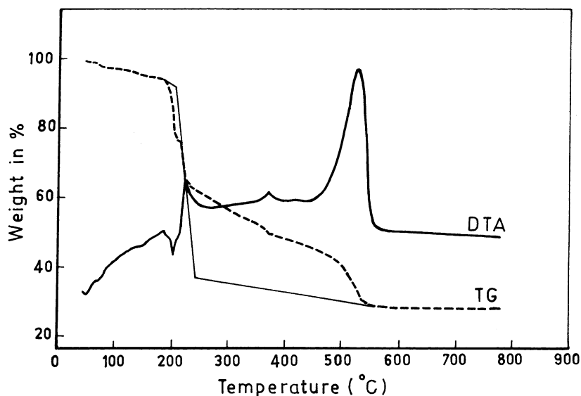
Fig. 3. TG–DTA of the complex (Dy 5 ).
