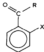
S- trans
