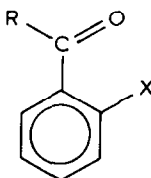
S- cis
