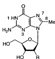
1a R = OH
