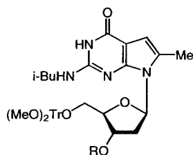
3a R = P(O)HO - Et 3 NH +
