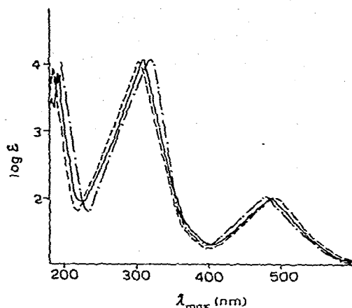
Fig. 1. The electronic spectra of (thioisobutyrylthio)trimethylsilane (----), -germane (—) and -tin (— · —).
