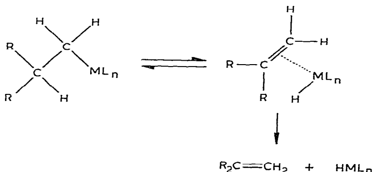
Fig. 1. β-Wasserstoff-Übertragung mit anschliessender Alken-Eliminierung.
